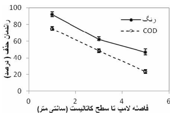
شکل ۹- تأثیر فاصله لامپ تا سطح کاتالیست در کاهش رنگ متیلن بلو و COD
