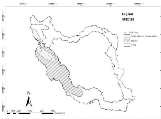
شکل ۳. نقشه پراکنش Quercus infectoria ۵- توالی‌های DNA هسته‌ای (ناحیه ITS)
