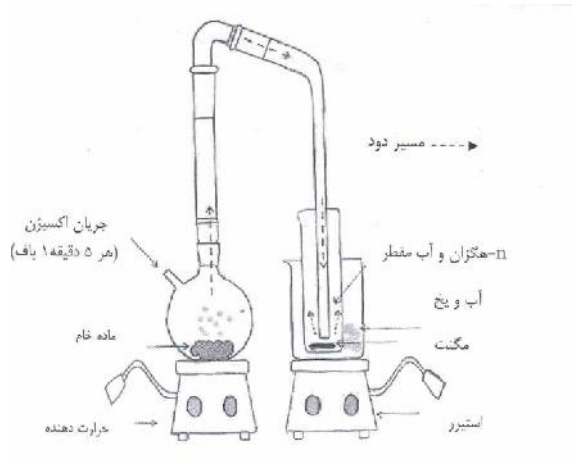
شکل ۱. شمایی از دستگاه طراحی شده و نحوه تولید و جمع آوری دود دارویی عنبر نسارا مطالعات بیولوژیک
