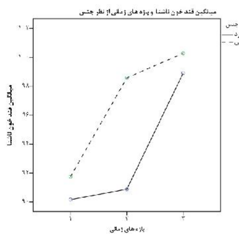
نمودار ۳. میانگین قند خون ناشتا و بازه های زمانی از نظر جنس
