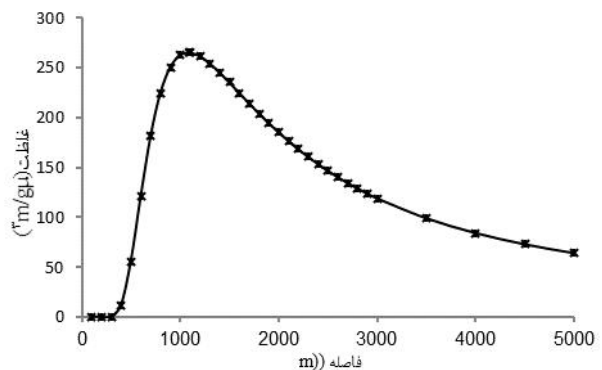
نمودار ۲. نحوه پراکنش SO_2 در شرایط خنثی و سرعت ۶\text{m/s}
