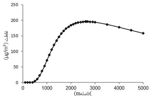
نمودار ۴. نحوه پراکنش NO_x در شرایط پایدار و سرعت ۴\text{m/s}
