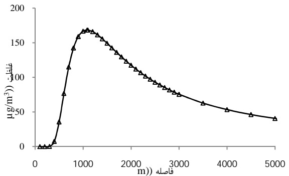
نمودار ۱. نحوه پراکنش NO_x در شرایط خنثی و سرعت ۶\text{m/s}
