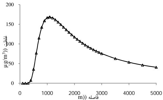
نمودار ۱. نحوه پراکنش NO_x در شرایط خنثی و سرعت 6\text{ m/s}
