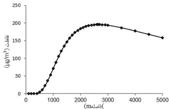
نمودار ۴. نحوه پراکنش NO_x در شرایط پایدار و سرعت 4\text{ m/s}
