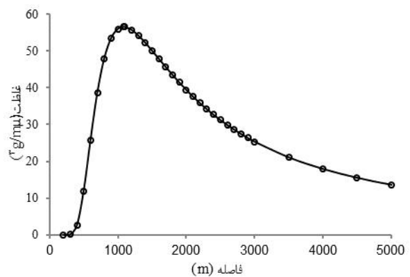
نمودار ۳. نحوه پراکنش ذرات PM در شرایط خنثی و سرعت 6\text{ m/s}
