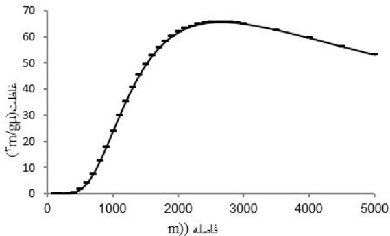
نمودار ۶. نحوه پراکنش PM در شرایط پایدار و سرعت ۴\text{m/s}
