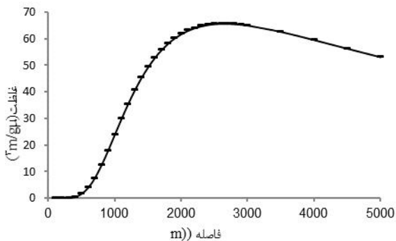
نمودار ۶. نحوه پراکنش PM در شرایط پایدار و سرعت 4\text{ m/s}
