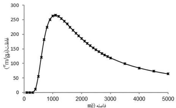
نمودار ۲. نحوه پراکنش SO_2 در شرایط خنثی و سرعت 6\text{ m/s}
