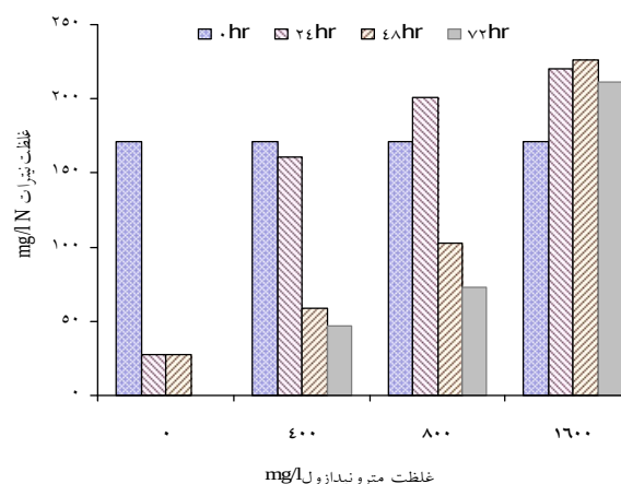
نمودار ۳- حذف ۱۷۱/۴۲ mg/l نیترات توسط باکتری سودوموناس استوتزری در حضور ۴۰۰، ۸۰۰ و ۱۶۰۰ mg/l مترونی‌دازول در دمای ۲۷°C و pH=۷/۲
