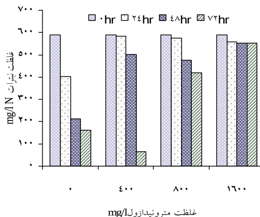
نمودار ۵- حذف ۵۹۰ mg/l نیترات توسط باکتری‌های سودوموناس استوتزری در حضور ۴۰۰، ۸۰۰ و ۱۶۰۰ mg/l مترونی‌دازول در دمای ۲۷°C و pH=۷/۲
