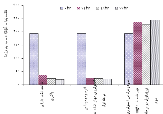
نمودار ۶- حذف ۱۹۴ mg/l نیترات توسط سودوموناس استوتزری طی دو مرحله تماس با ۸۰۰ mg/l مترونی‌دازول
