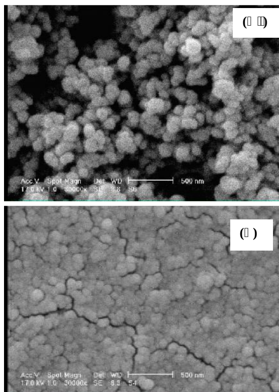
شکل ۳. تصویر میکروسکوپی روبشی از الف) نانو ذرات اکسیدروی تثبیت شده روی شیشه (ب) نانو ذرات اکسیدروی به همراه نانو ذرات سیلیس (۱۰٪) تثبیت شده روی شیشه
