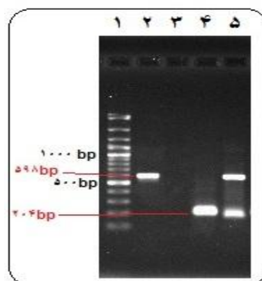
شکل ۱. نتایج ژل الکتروفورز محصولات Duplex PCR نمونه‌های BAL: چاهک ۱: مارکر (DNA Ladder, SM#333, ۱۰۰bp)، چاهک ۲: کنترل مثبت با جفت پرایمر NG، چاهک ۳: کنترل منفی، چاهک ۴: محصول PCR نمونه BAL سالم با پرایمر Bet و چاهک ۵: محصول Duplex نمونه BAL آلوده به گونه‌های نوکاردیا با پرایمر NG و Bet.
