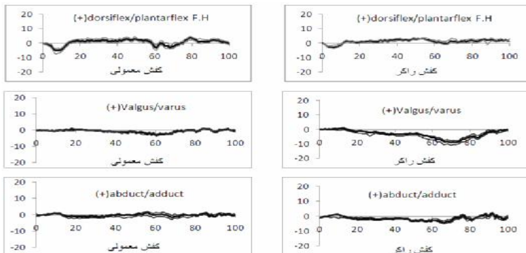
شکل شماره 4- نمایش حرکات سگمان قدامی نسبت به سگمان خلفی-میانی در طول یک سیکل راه رفتن در صفحات ساژیتال، فرونتال و عرضی هنگام استفاده از کفش راکر و معمولی
