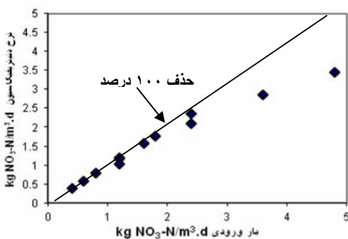
شکل ۷- نرخ‌های دنیتریفیکاسیون برای مقادیر مختلف بارگذاری نیترات ( 4/8-4/4 \text{kgNO}_3\text{-N/m}^3\text{.d} ) در ۴ نوبت کاری پایلوت (غلظت‌های نیترات ورودی ۲۰۰-۵۰)
