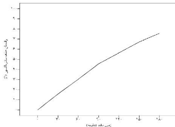
شکل ۲. تغییرات میانگین درصد حذف سفتریاکسون در زمان‌های ماند مختلف ( \text{H}_2\text{O}_2=15\text{mg/l} , \text{pH}=3 ، شدت تابش لامپ \text{UV}=36 وات و غلظت اولیه آنتی بیوتیک =9\text{ mg/l} )
