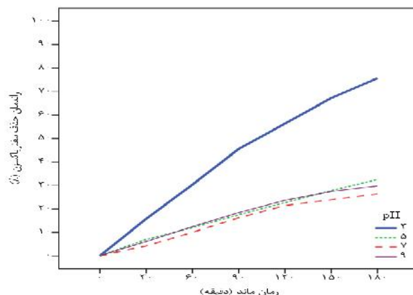
شکل ۳. تغییرات میانگین درصد حذف سفتریاکسون در زمان‌های ماند مختلف و pH های متفاوت ( \text{H}_2\text{O}_2=15\text{mg/l} ، شدت تابش لامپ \text{UV}=36 وات و غلظت اولیه آنتی بیوتیک =9\text{ mg/l} )
