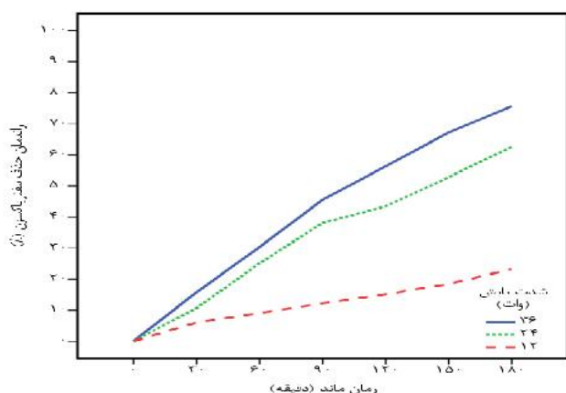
شکل ۵. تغییرات میانگین درصد حذف سفتریاکسون به تفکیک شدت تابش UV و زمان‌های ماند مختلف (غلظت اولیه آنتی بیوتیک =9\text{ mg/l} ، \text{H}_2\text{O}_2=15\text{mg/l} ، \text{pH}=3 )
