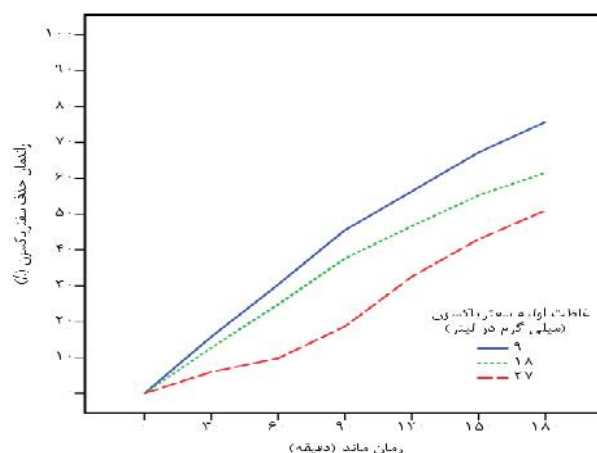
شکل ۶. تغییرات میانگین درصد حذف سفتریاکسون به تفکیک غلظت‌های اولیه مختلف آنتی بیوتیک سفتریاکسون و زمان‌های ماند مختلف ( H_2O_2=5mg/l ، pH=3 ، شدت تابش UV=36 وات)
