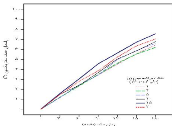
شکل ۴. تغییرات میانگین درصد حذف سفتریاکسون در غلظت‌های مختلف \text{H}_2\text{O}_2 و زمان‌های ماند متفاوت ( \text{pH}=3 ، شدت تابش لامپ \text{UV}=36 وات و غلظت اولیه آنتی بیوتیک =9\text{ mg/l} )
