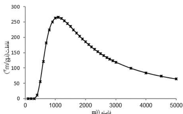
نمودار ۲. نحوه پراکنش \text{SO}_2 در شرایط خنثی و سرعت ۶ m/s
