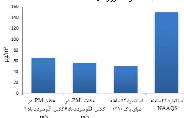
نمودار ۹. مقایسه حداکثر غلظت \text{PM} پیش بینی شده توسط SCREEN3 با استاندارد کشور و NAAQS
