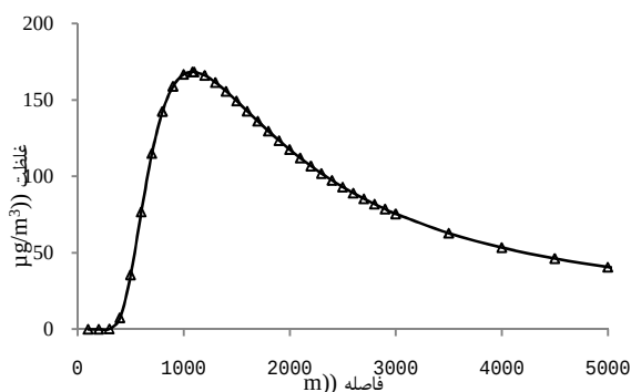
نمودار ۱. نحوه پراکنش \text{NO}_x در شرایط خنثی و سرعت ۶ m/s
