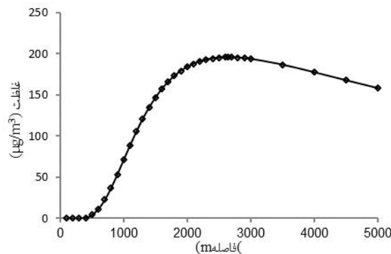
نمودار ۴. نحوه پراکنش \text{NO}_x در شرایط پایدار و سرعت ۴ m/s
