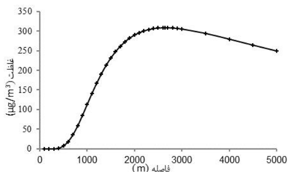
نمودار ۵. نحوه پراکنش \text{SO}_2 در شرایط پایدار و سرعت ۴ m/s
