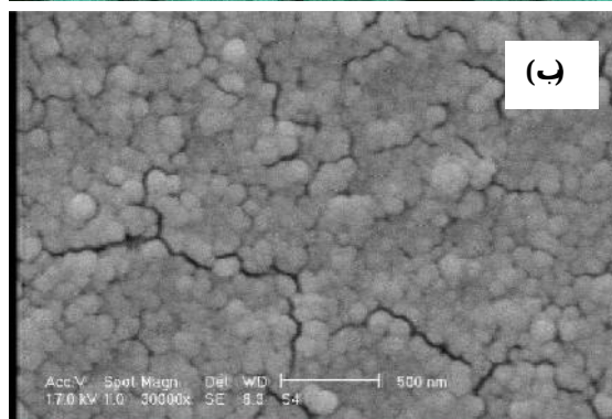
شکل ۳. تصویر میکروسکوپی روبشی از (الف) نانو ذرات اکسیدروی تثبیت شده روی شیشه (ب) نانو ذرات اکسیدروی به همراه نانو ذرات سیلیس (۱۰٪) تثبیت شده روی شیشه
