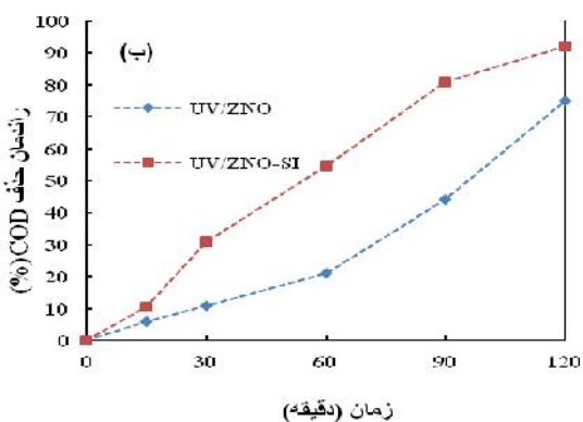
شکل ۵. مقایسه دو سیستم UV/ZnO و UV/Silica-ZnO در (الف) بازدهی رنگبری متیلن بلو و (ب) حذف COD (غلظت رنگ: ۲۵ میلی گرم در لیتر، شدت تابش: ۳۹۵۰ میکرووات بر سانتی متر مربع، pH=۷، فاصله یک سانتی متری لامپ تا سطح کاتالیست)
