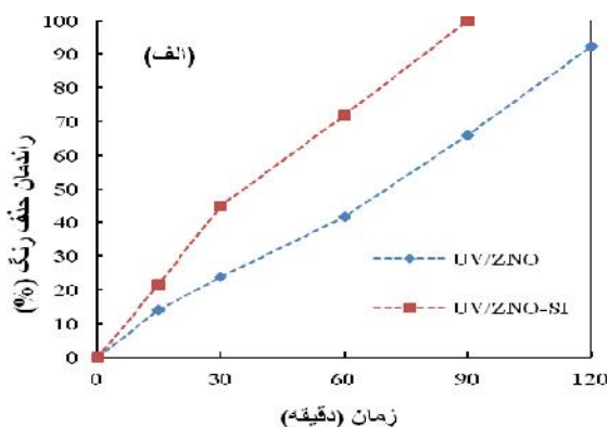
شکل ۴. تأثیر درصد سیلیس بر میزان (الف) رنگبری متیلن بلو با سیستم UV/Silica-ZnO (ب) حذف COD متیلن بلو با سیستم UV/Silica-ZnO (غلظت رنگ: ۲۵ میلی گرم در لیتر، شدت تابش: ۳۹۵۰ میکرووات بر سانتی متر مربع، pH=۷، فاصله یک سانتی متری لامپ تا سطح کاتالیست)
