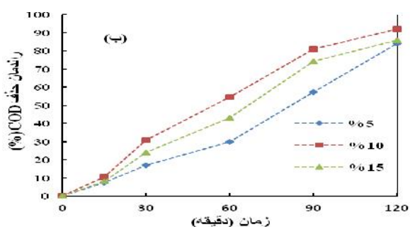
شکل ۴. تأثیر درصد سیلیس بر میزان (الف) رنگبری متیلن بلو با سیستم UV/Silica-ZnO (ب) حذف COD متیلن بلو با سیستم UV/Silica-ZnO (غلظت رنگ: ۲۵ میلی گرم در لیتر، شدت تابش: ۳۹۵۰ میکرووات بر سانتی متر مربع، pH=۷، فاصله یک سانتی متری لامپ تا سطح کاتالیست)
